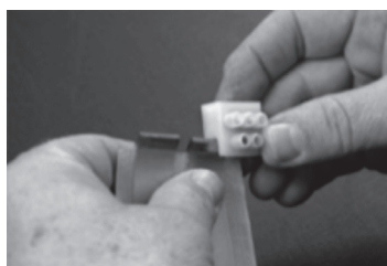
Figura 20 – Encaixar o conector de 3 saídas deslizando-o lateralmente
